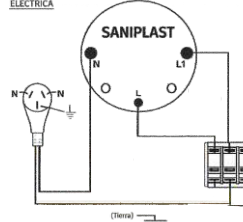
DIAGRAMA DE CONEXION ELECTRICA
